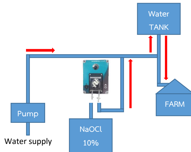
รูปที่ 1 แสดงวิธีการติดตั้งเครื่อง Cl-800 Fig. 1 Install a Cl-800.
