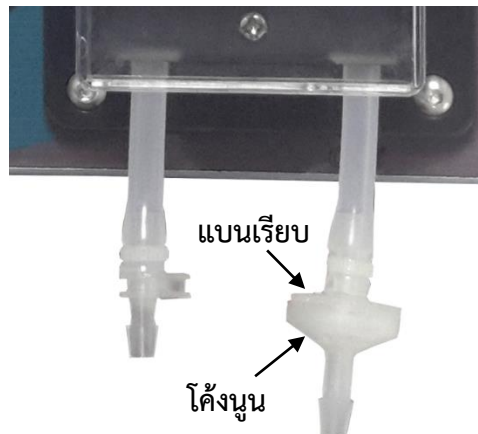
รูปที่ 4 แสดงลักษณะทางเข้า-ทางออก ของซีควาล์ว Fig. 4 Check Valve (One way valve)
